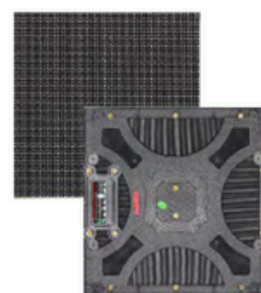
P4.81-13S MODULE
