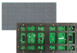
P6.67-6S MODULE
